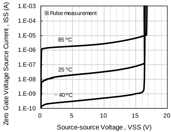
ISS - VSS
